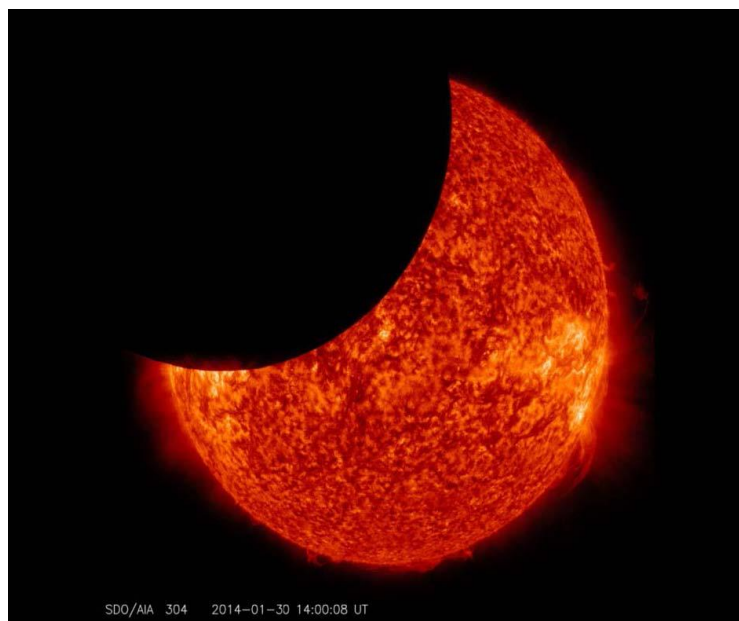
Eclipse partielle de Soleil vue depuis l'espace / Mission SDO / Source : Nasa
